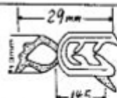
LHCW0052 DOOR WEATHER STRIP
